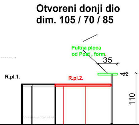
Pogled B
