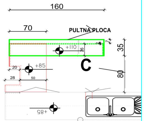
Pogled C
