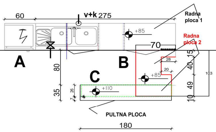
Pogled A
