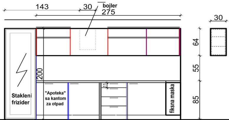
Pogled A
