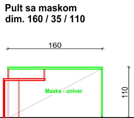
Pogled C
