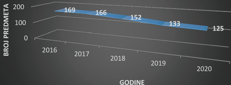
Prikaz trenda smanjenja broja neriješenih predmeta ratnih zločina u sudovima
