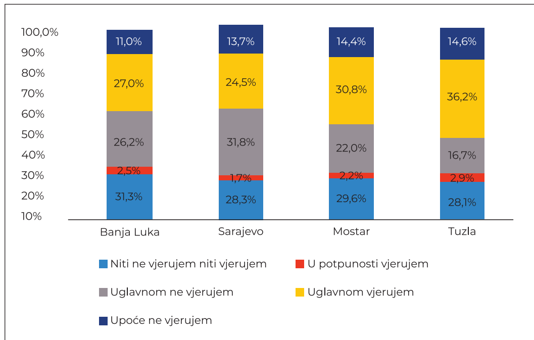
GRAFIKON 5. OPĆI STUPANJ POVJERENJA U SUDOVE BiH
